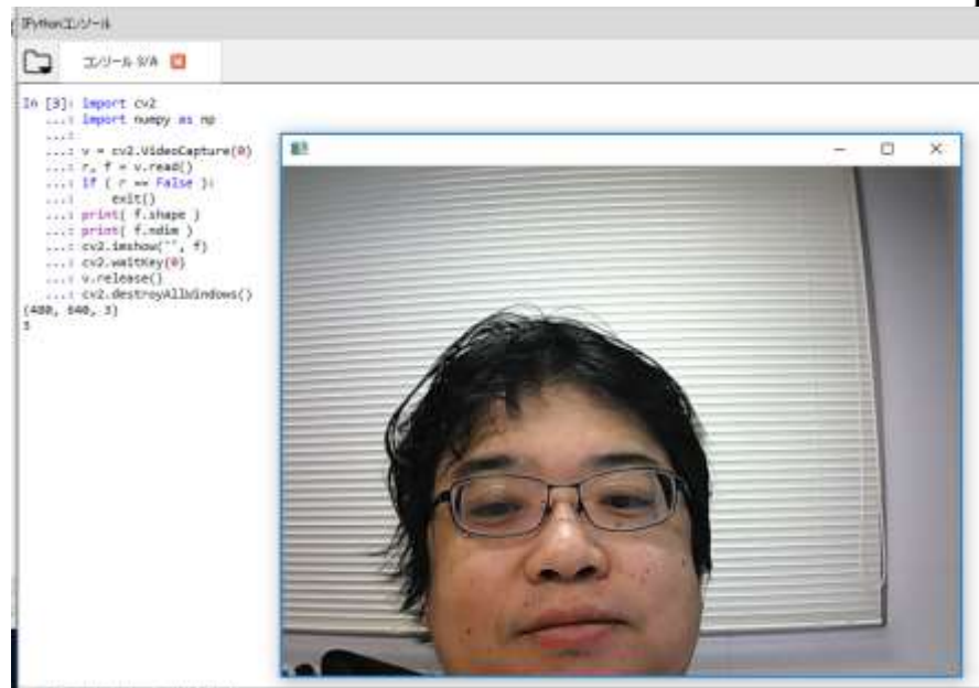
動作画面
